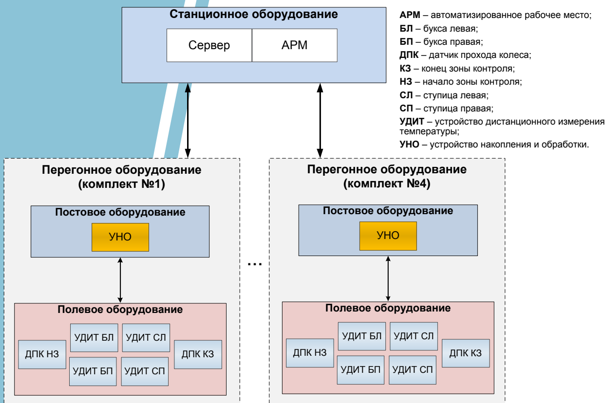
Структура АКРО-Б
