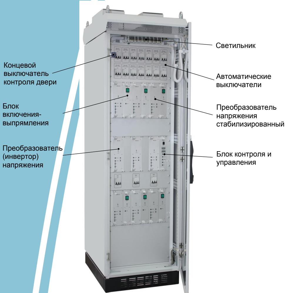
Шкаф гарантированного питания ШГПЛ-1
