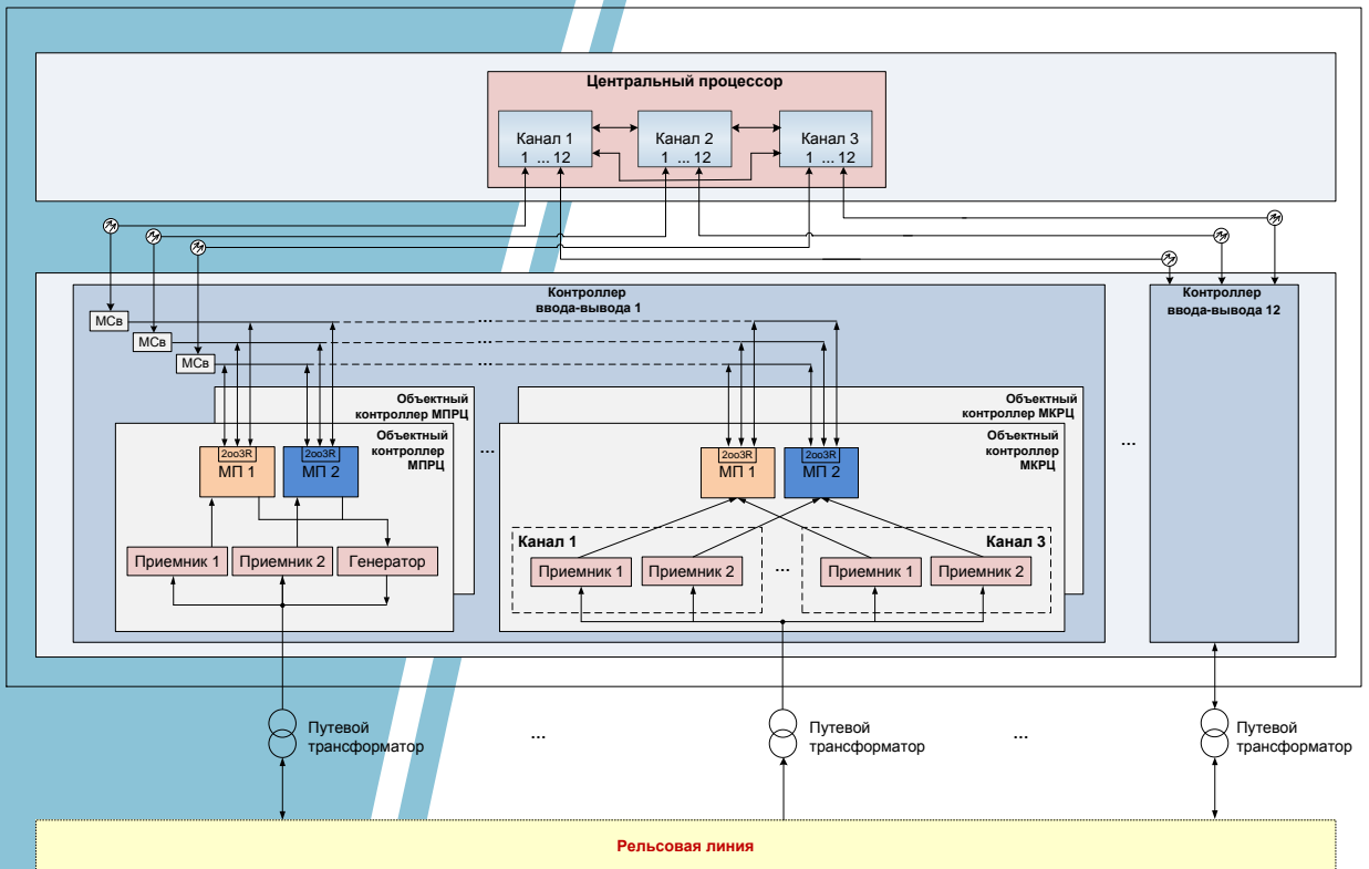
Структура МРЦ-У
