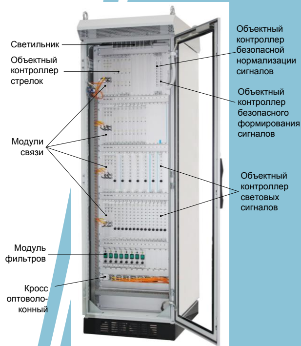
ШКиУ без центрального процессора
